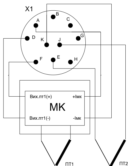
Рисунок В.3г – Електрична схема приєднання ПТК-01 АС 2ХА(К)-МК, ПТК-01 АС 2НН(Н)-МК
