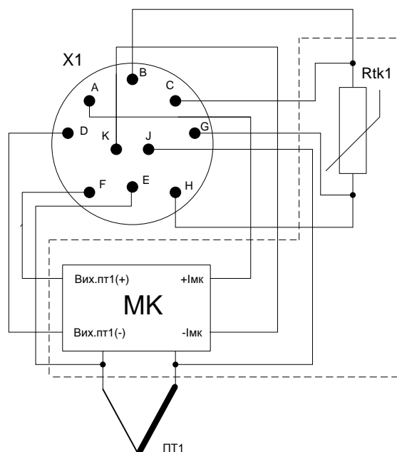
Рисунок В.8д – Електрична схема приєднання ПТК-01 АС 1ХА(К)-МК-1ТОП, ПТК-01 АС 1НН(Н)-МК-1ТОП
